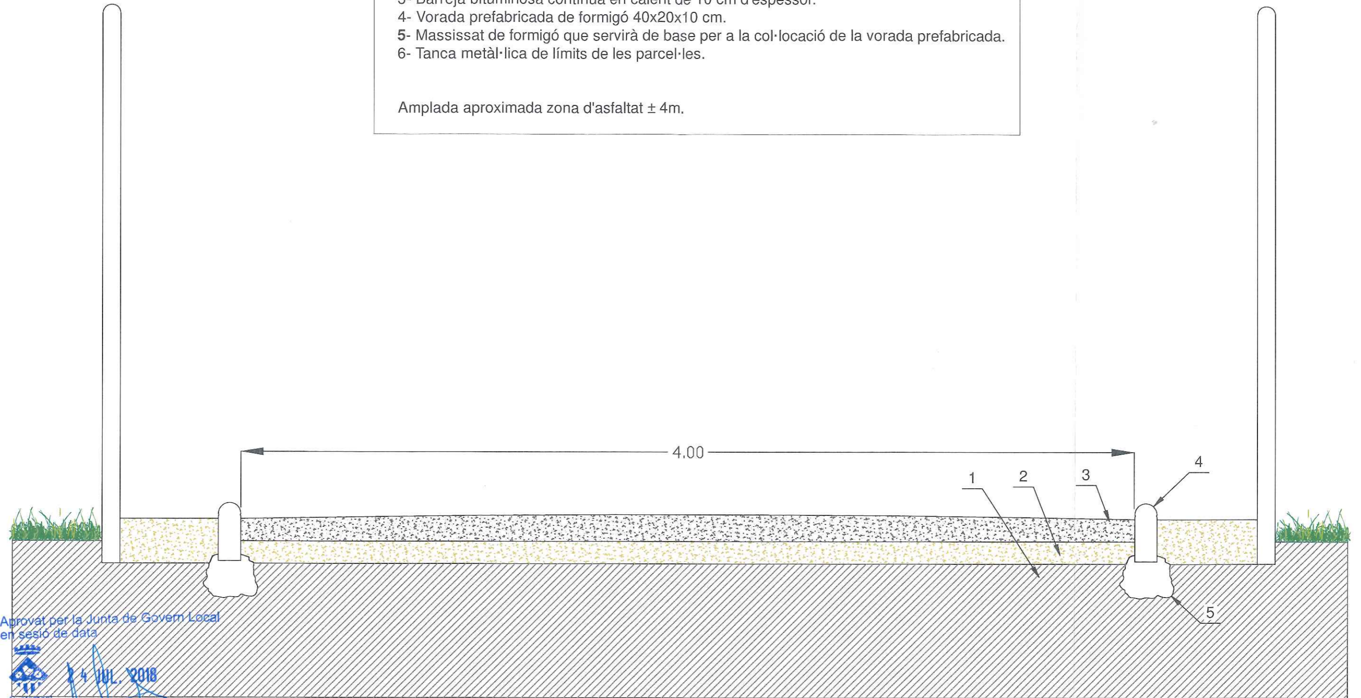
Detall de Secció tipus
