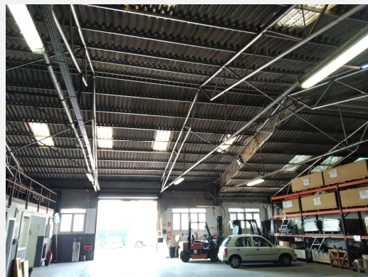
Foto 7. Detall coberta
